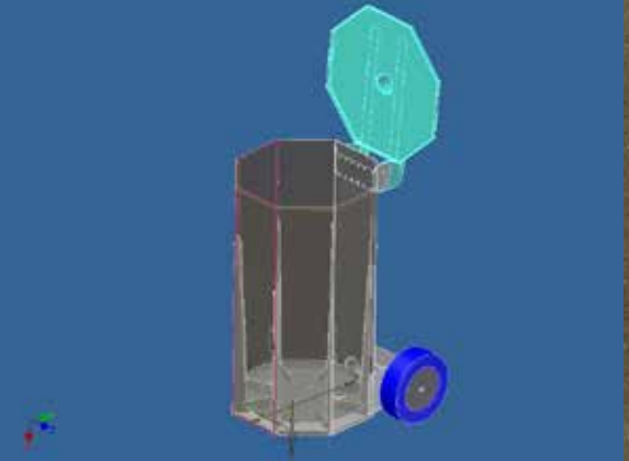
Absaugtonne
